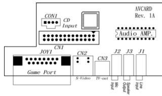
AV Card
